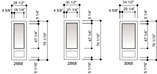
Hinged Patio Door - Inswing
